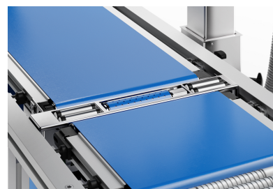
Ленточный аппликатор
