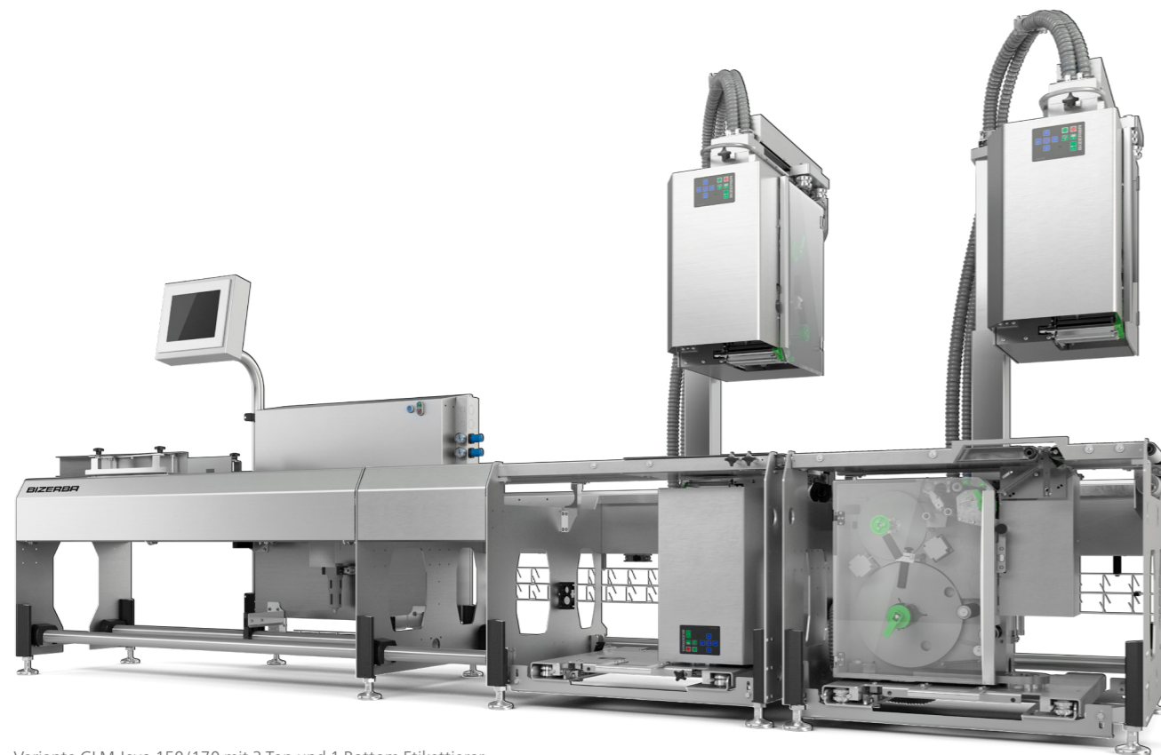
Variante GLM-levo 150/170 mit 2 Top und 1 Bottom Etikettierer
